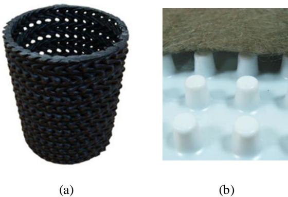
圖 10. 地工網管(a)及地工排水板(b)
