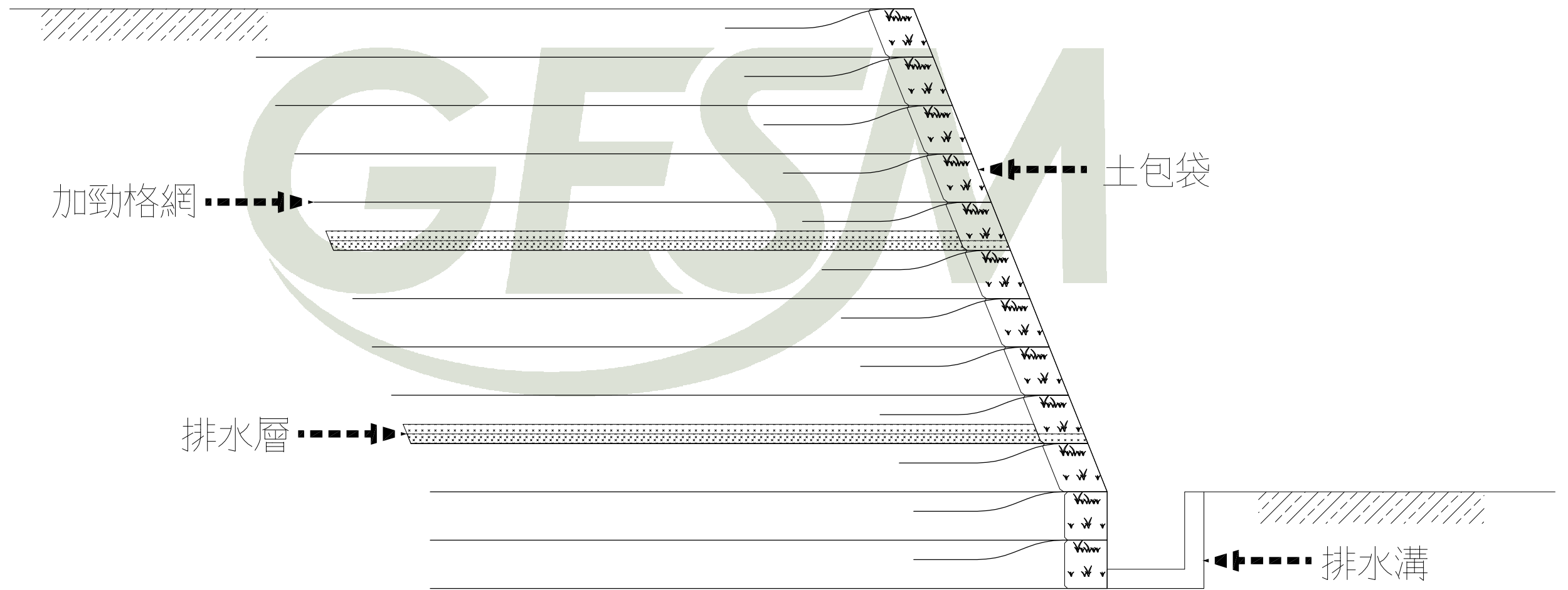
回包式加勁擋土牆示意圖
