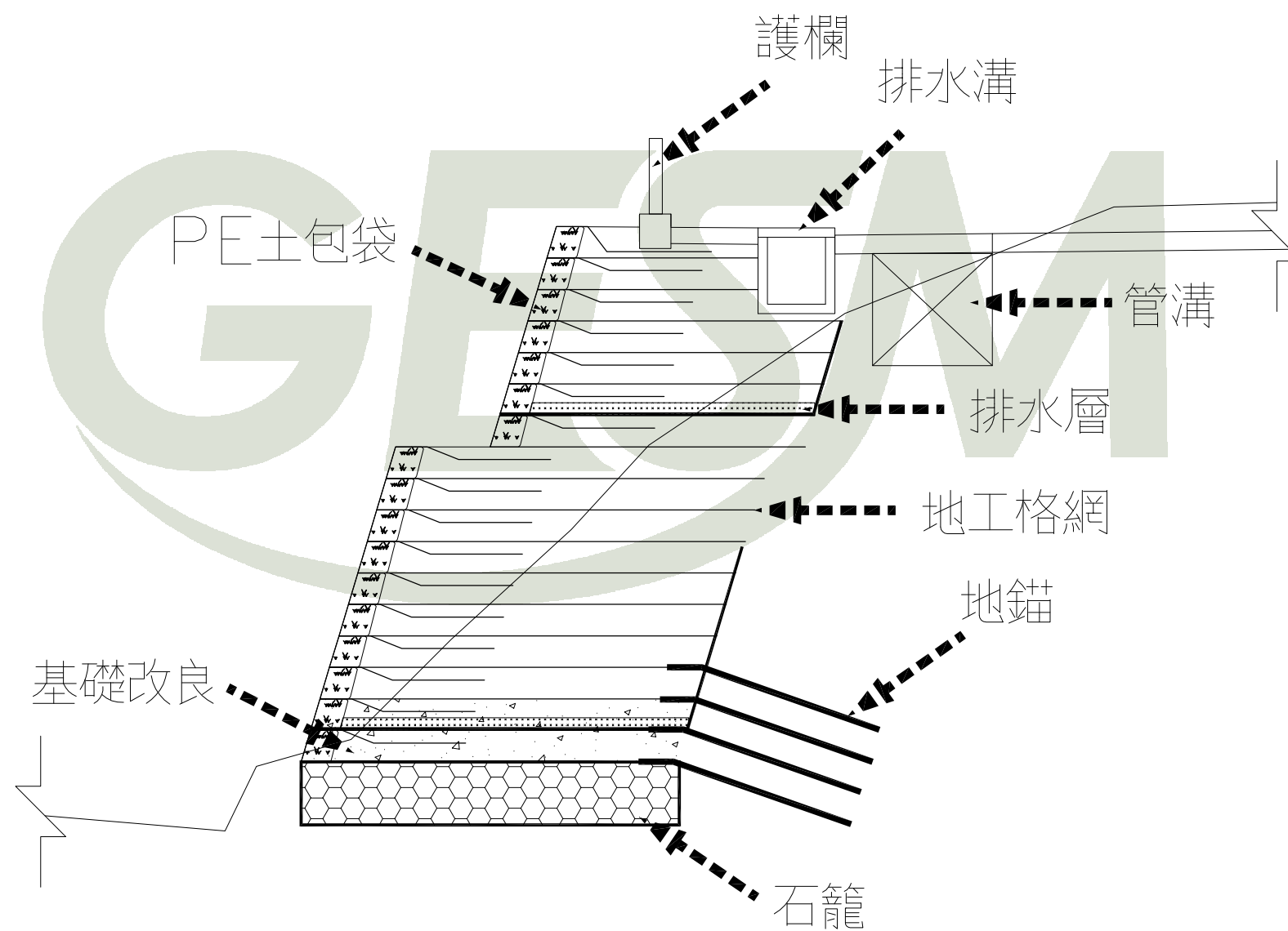
回包式加勁擋土牆及石籠示意圖
